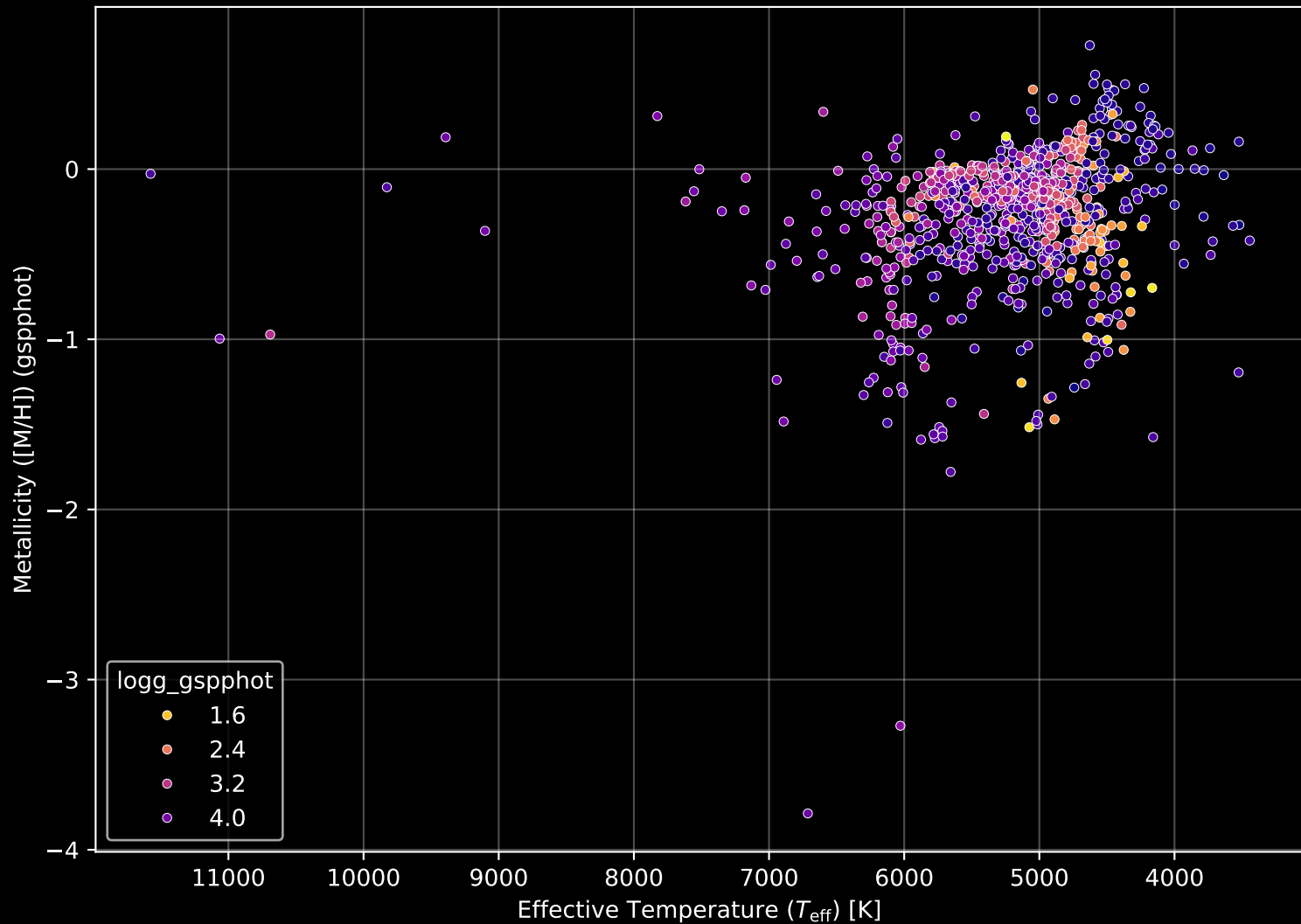
APOGEE DR17 Field: [M15] Stellar Population Parameters (n= 926)
